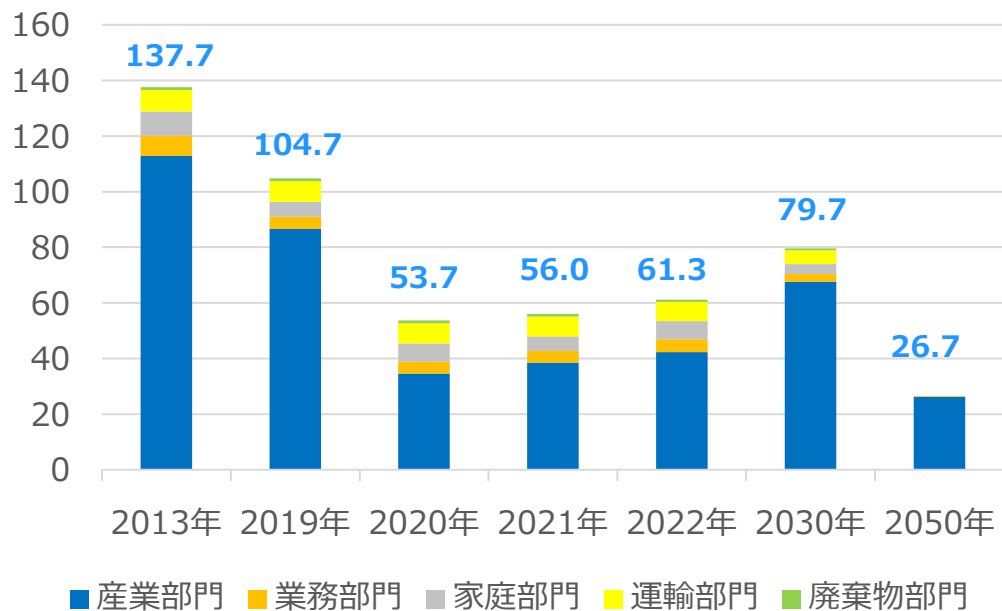
部門別排出量の推移（単位：万t-CO2）
