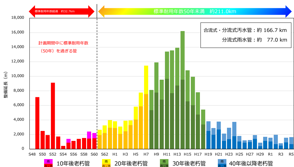
図 3.3-2 布設年度別管路延長（令和 5（2023）年度現在）
