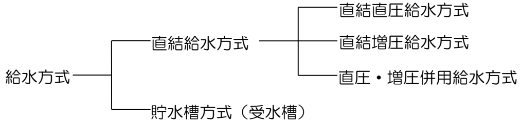
図5-1 給水方式
