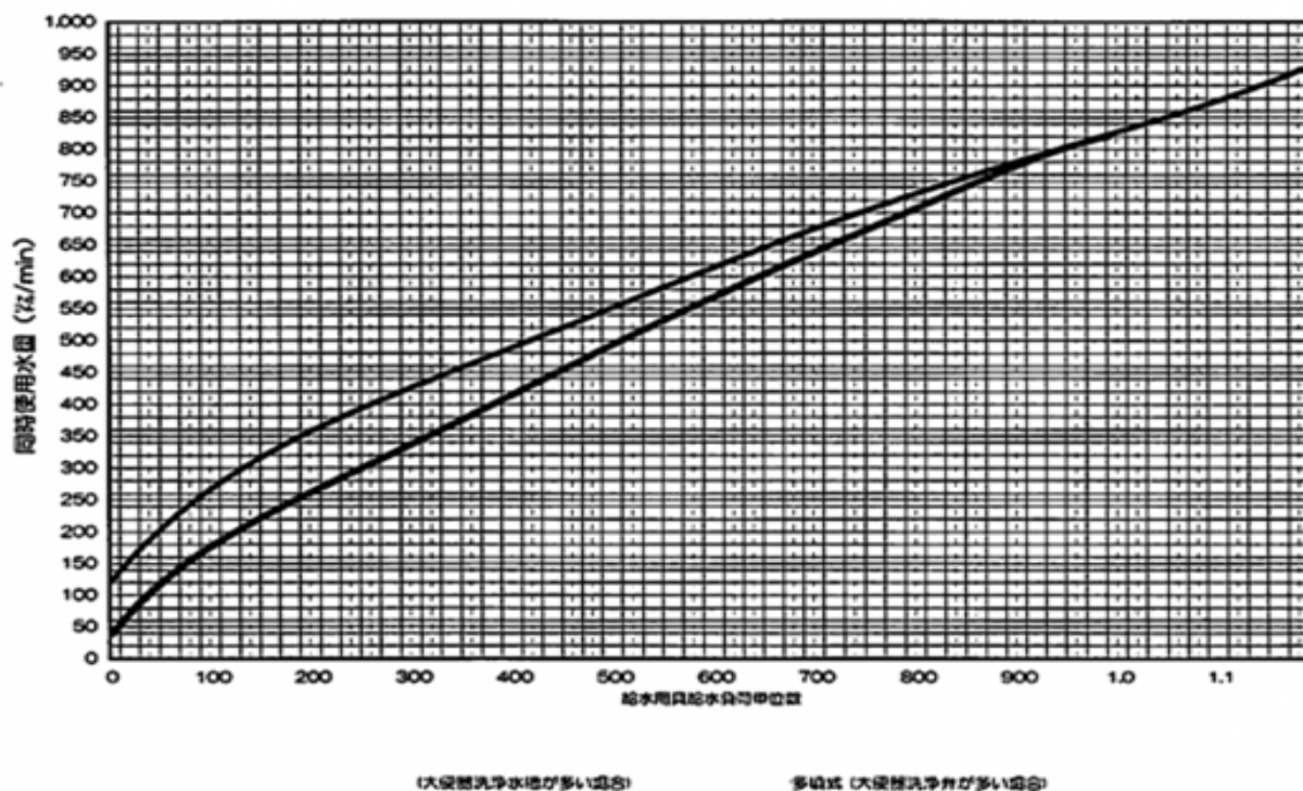
図7-4 同時使用水量－器具給水負荷単位関係図（Hunter曲線）
