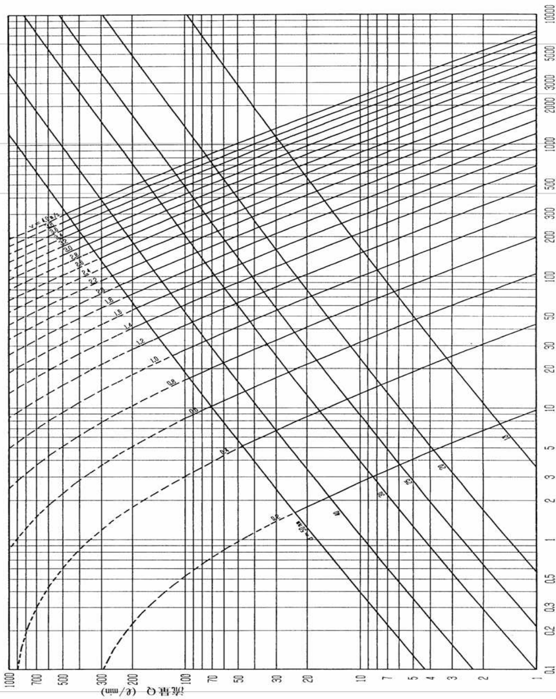
動水分配 I (%) ウエストン公式流量図表
