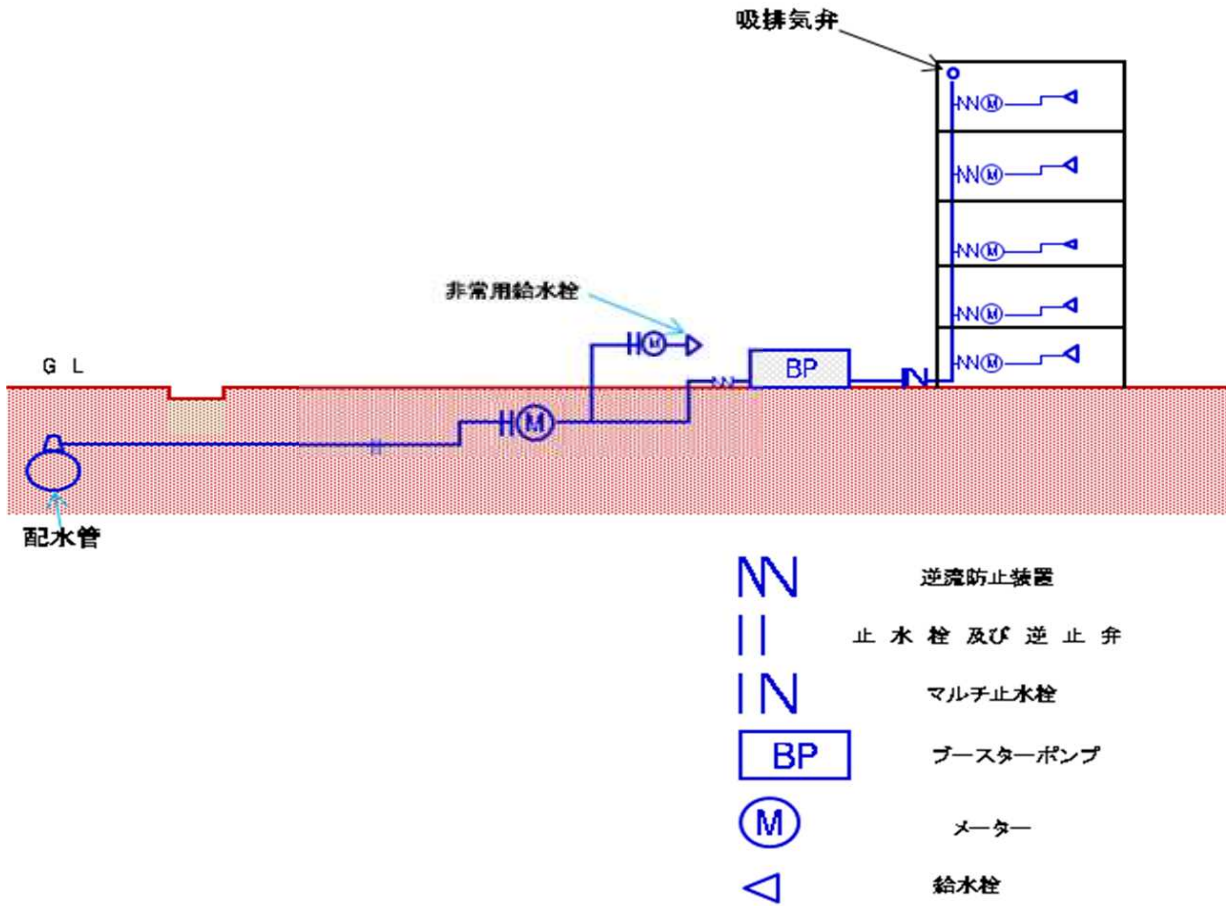
図5-5 直圧・増圧併用給水方式
