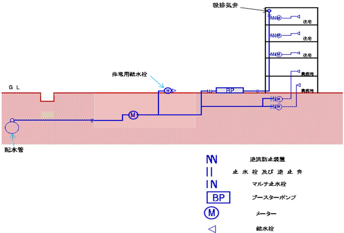
図5-5 直圧・増圧併用給水方式
