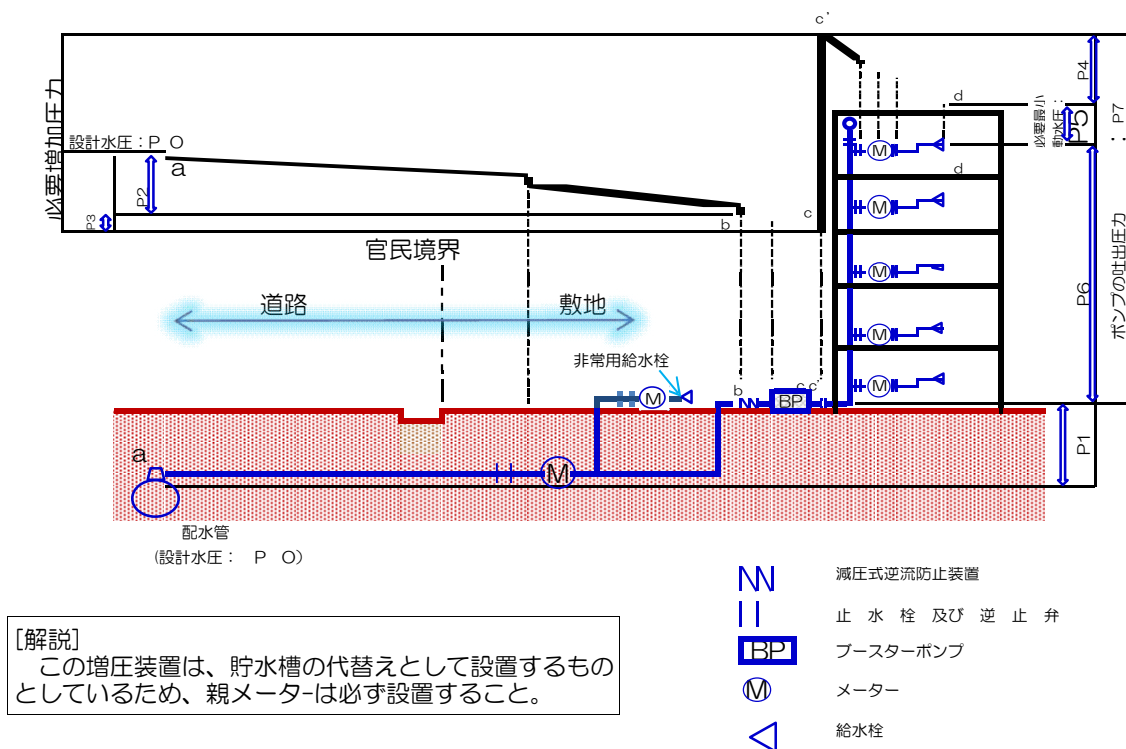
図7-1 直結増圧給水方式による動水勾配図
