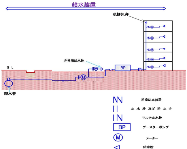
図5-3 直結増圧式の場合
