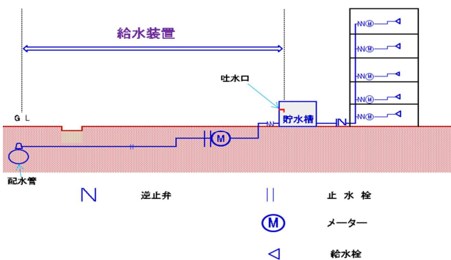
図5-2 貯水槽の場合
